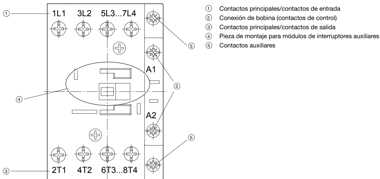
Figura 9: Esquema básico de contactor 4P
