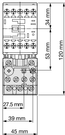
Figura 35: EVBxxxA
