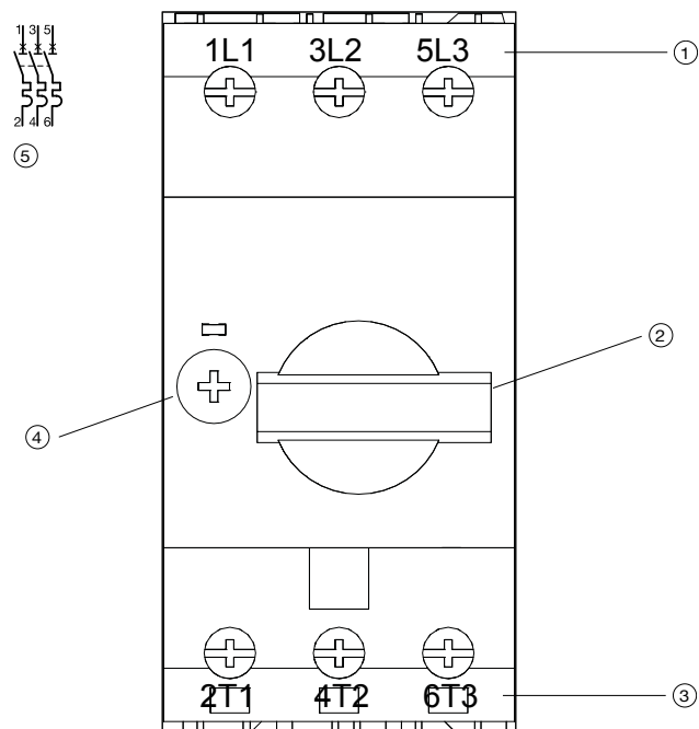
Figura 10: Esquema básico de guardamotor
