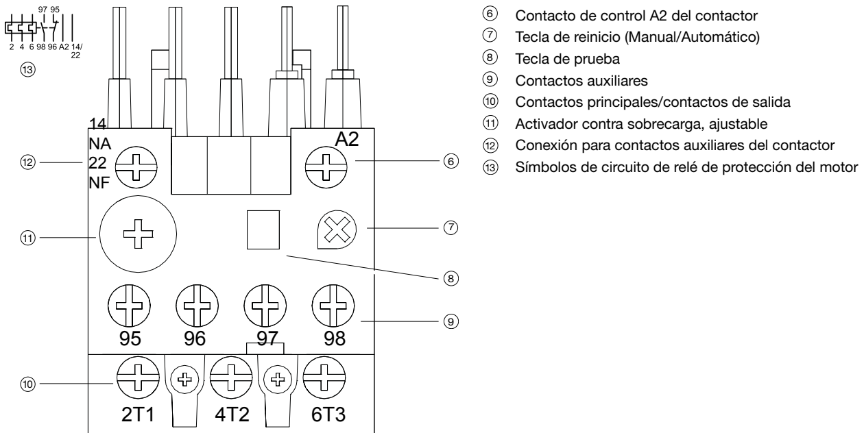
Figura 11: Esquema básico de un relé de protección del motor
